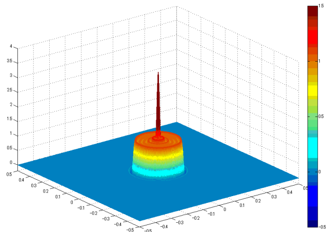
図2 Pinsky 現象
