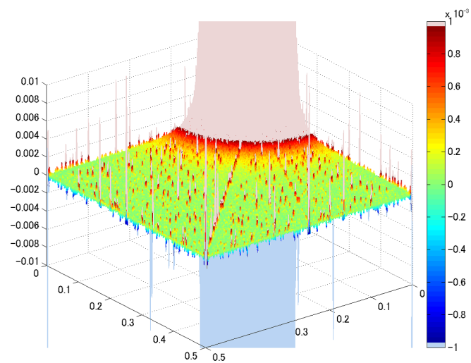
図5 倉坪現象 3
