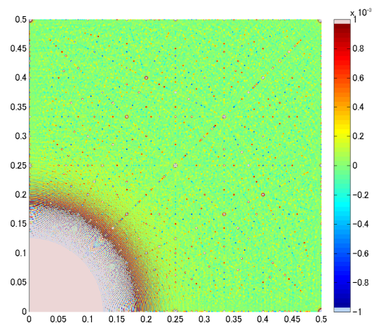
図6 倉坪現象 4
